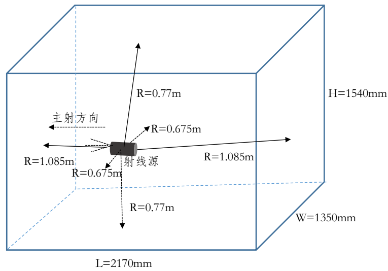
图 11-1 射线照射示意图
