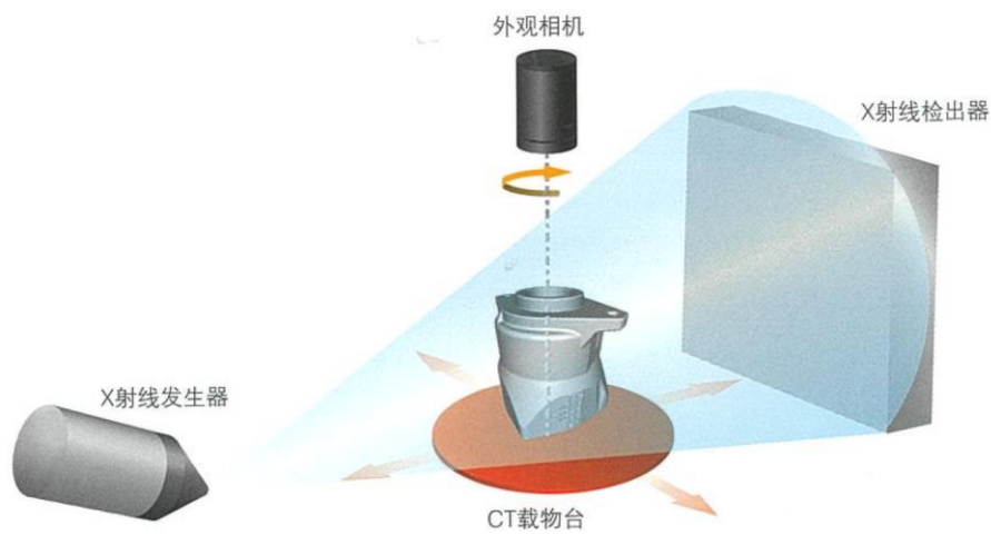
图 9-3 装置外观结构图
