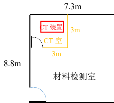
图 1-3 材料检测室、CT 室平面布置图
