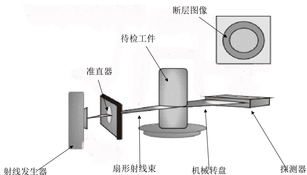
图 9-2 工业 CT 工作示意图
