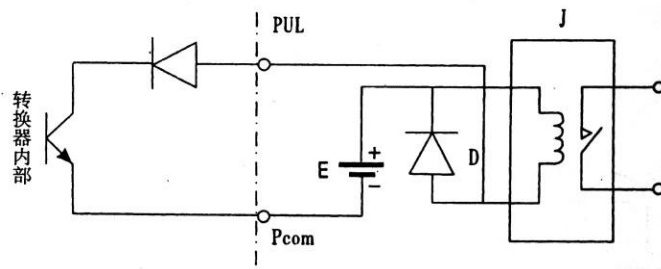
图十三 (c) 电子计数器接线
