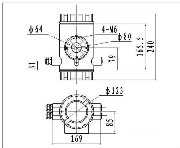
412B (蓝色) 圆表尺寸图
