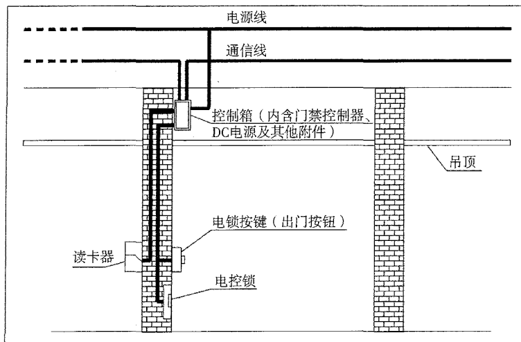
图8 出入口控制设备安装管线示意图
