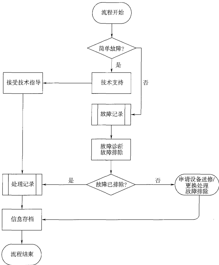
图 12 安全防范系统故障处理工作程序
