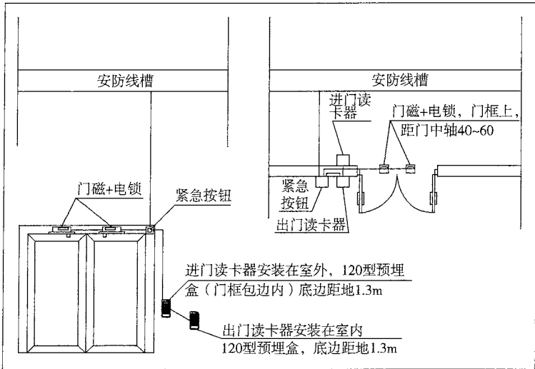
图9 双扇门双向控制玻璃门出入口控制设备安装示意图
