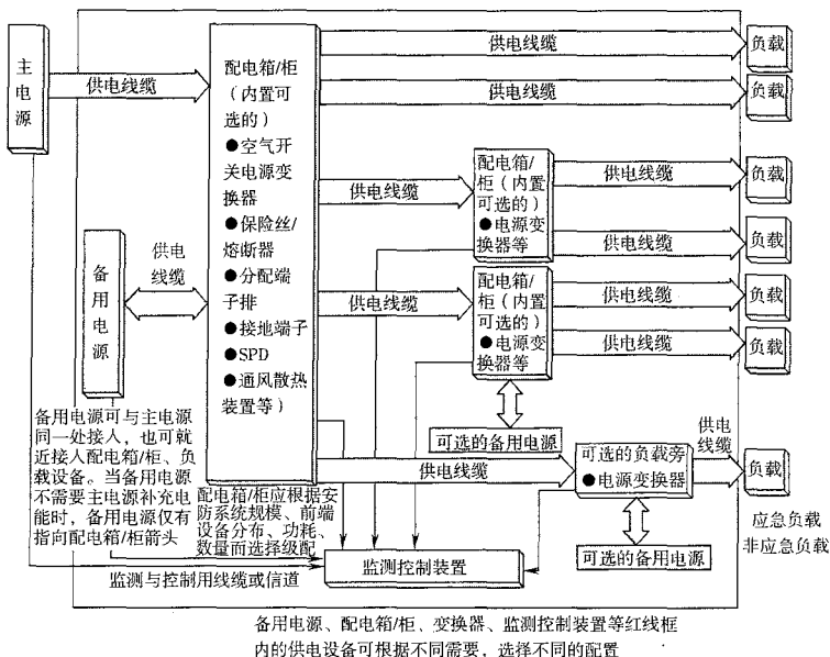
图 7 安全防范系统供电系统构成示意图
