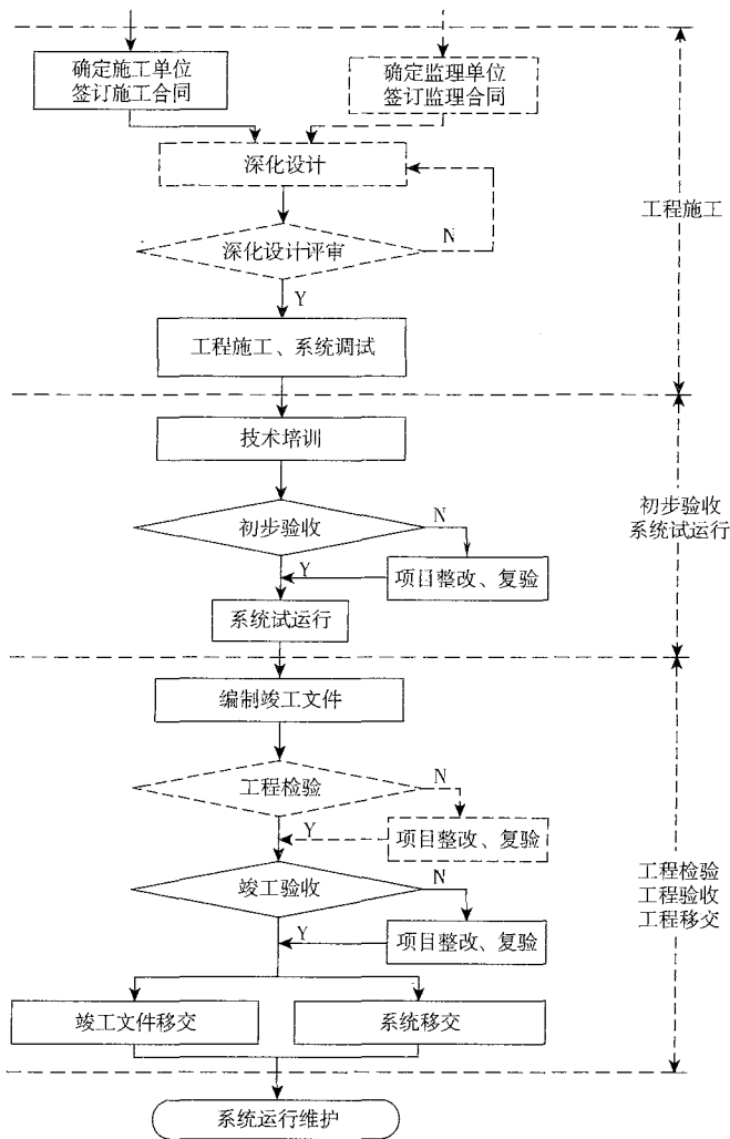
图2 安全防范工程建设程序示意图(续)
