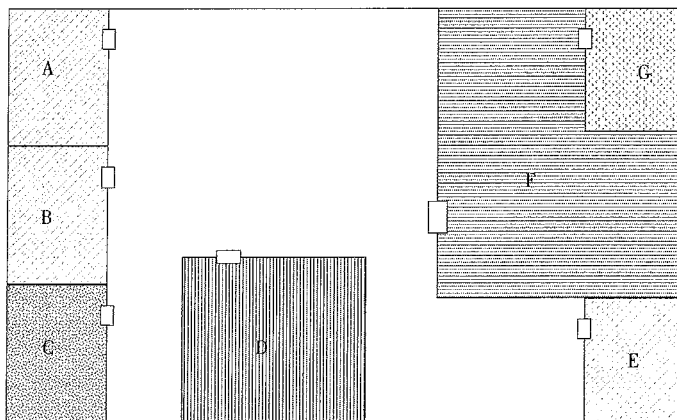
图 3 出入口控制系统受控区示意图
