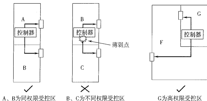
图 4 出入口控制系统受控区的设备安装示意图
