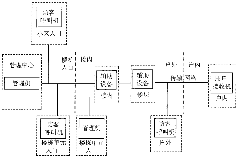
图 6 楼寓对讲系统应用构成示意图
