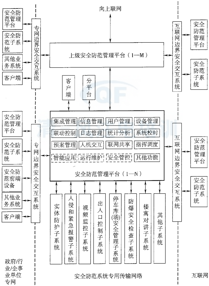
图 1 安全防范系统集成联网架构图
