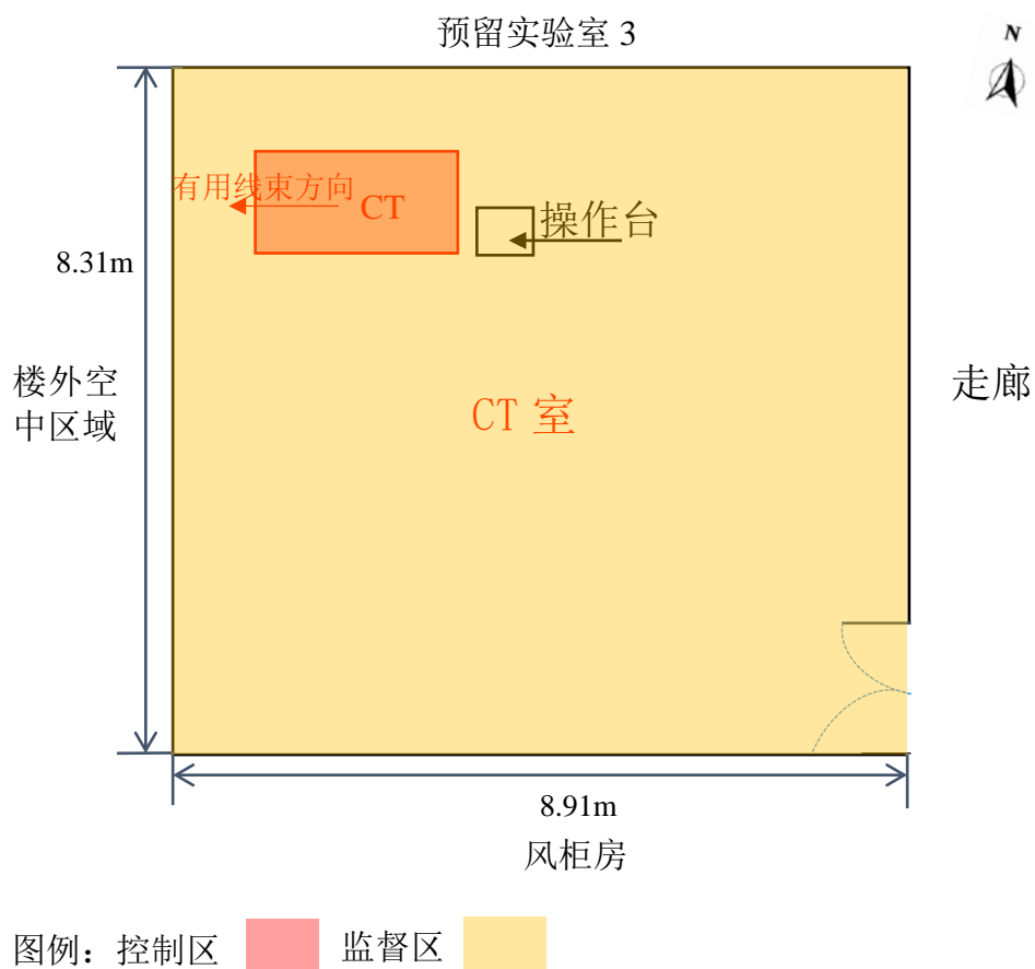
图 10-5 工作场所布局和分区示意图
