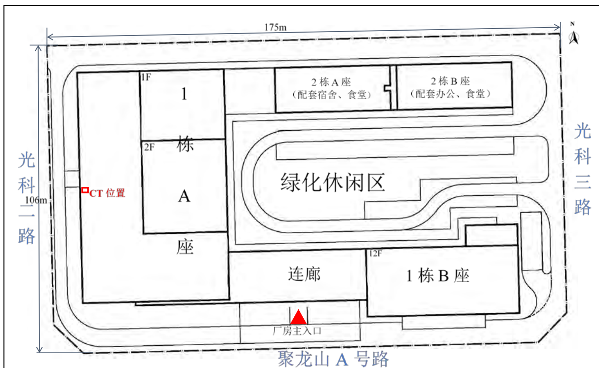
图 1-2 贝特瑞公司厂区平面布置图
