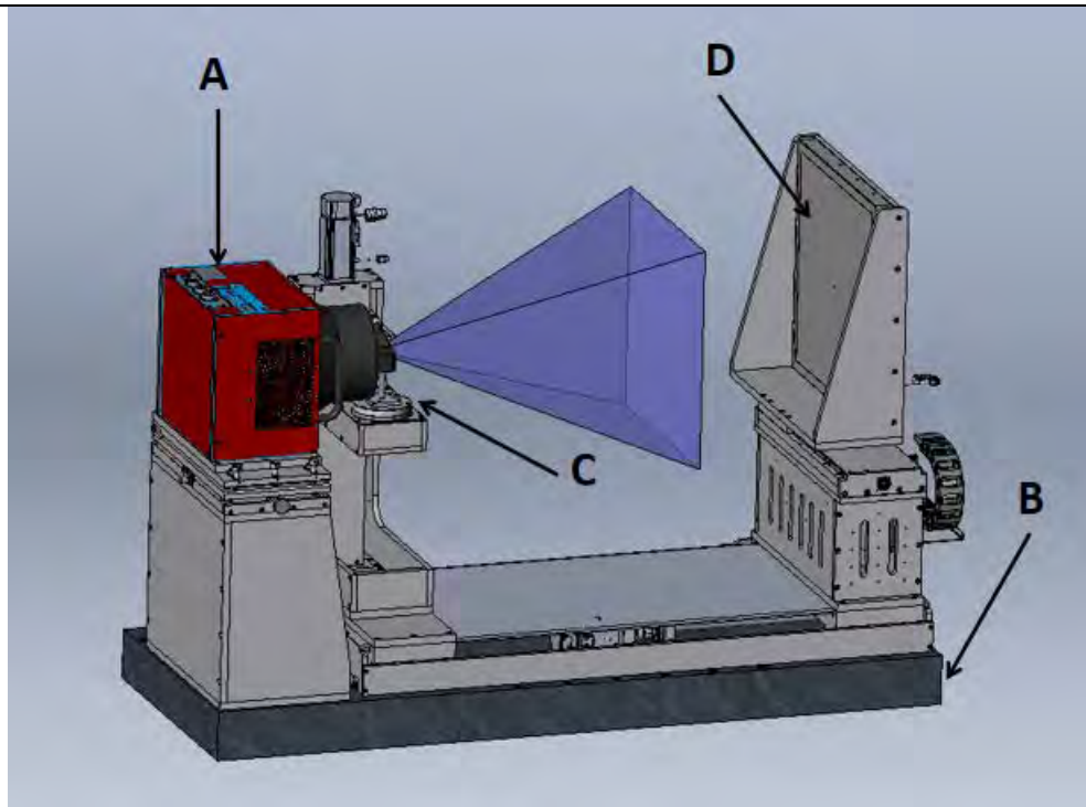
图 9-2 工业 CT 内部结构图
