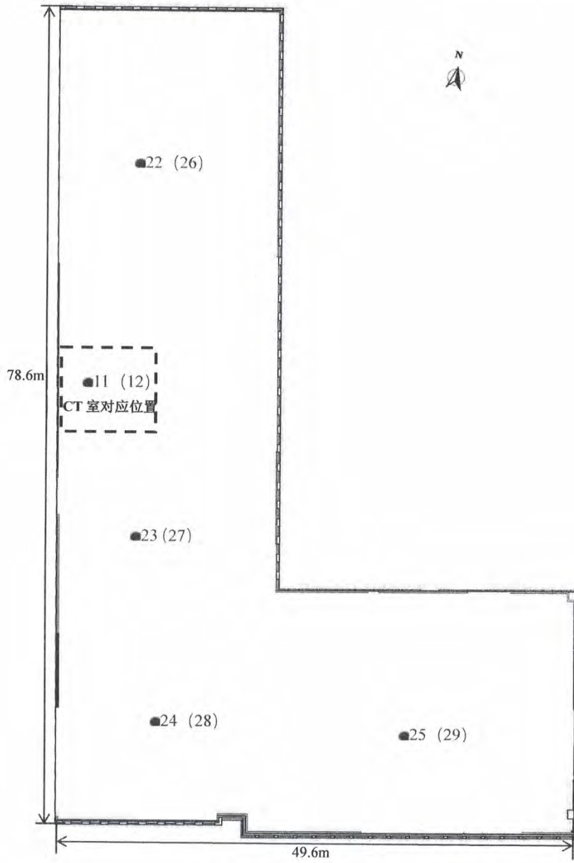
1 栋 A 座三（五）层布点示意图
