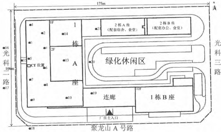
厂区布点示意图
